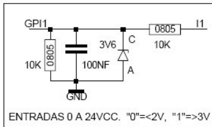
CIRCUITO EQUIVALENTE ENTRADAS
