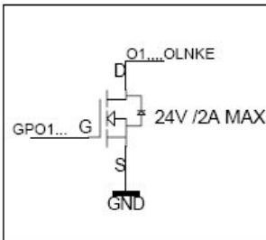
CIRCUITO EQUIVALENTE SALIDAS
